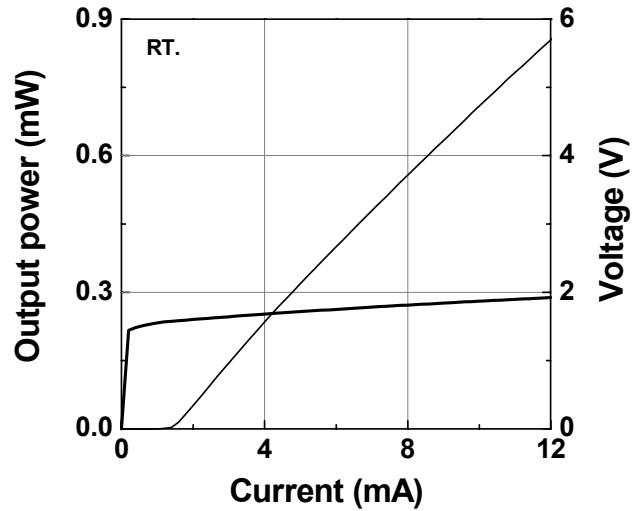
LIV Curve
